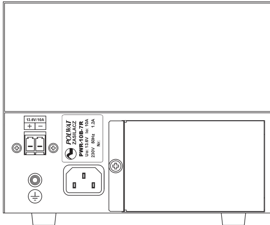
Rys.2. Panel przyłączeniowy zasilacza PWR-10B-7R
