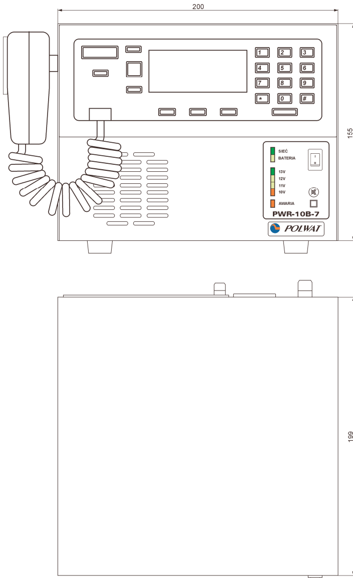
Rys.4. Wymiary gabarytowe zasilacza PWR-10B-7R
