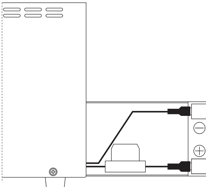
Rys.3. Wymiana akumulatora
